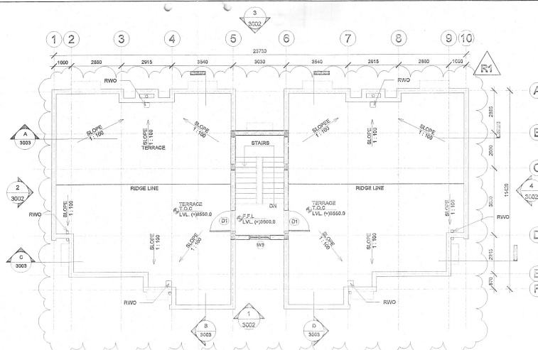
3 TERRACE PLAN 1:100
